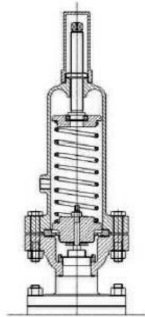
Actuator 140
