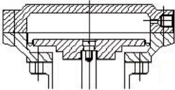
Actuator 245
